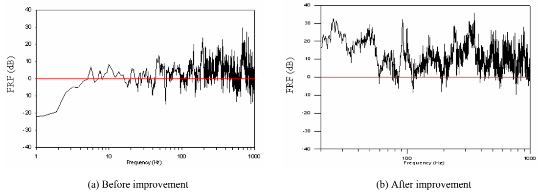
Fig. 13. Vibration isolation via mount A.
